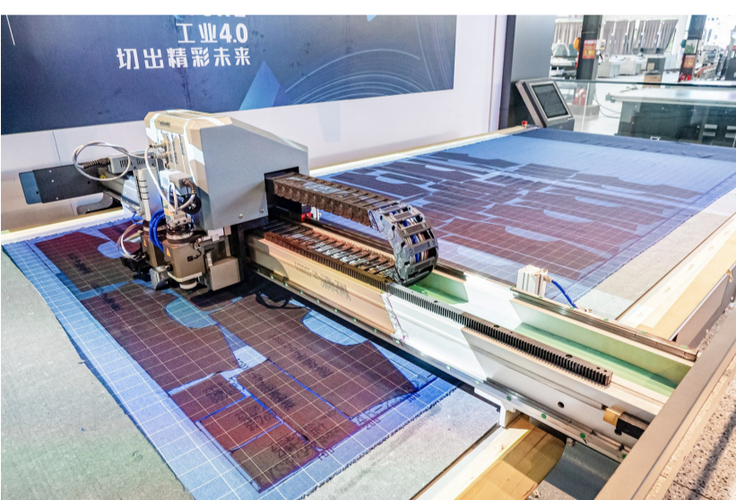
瑞洲科技切割机器人在工作。
