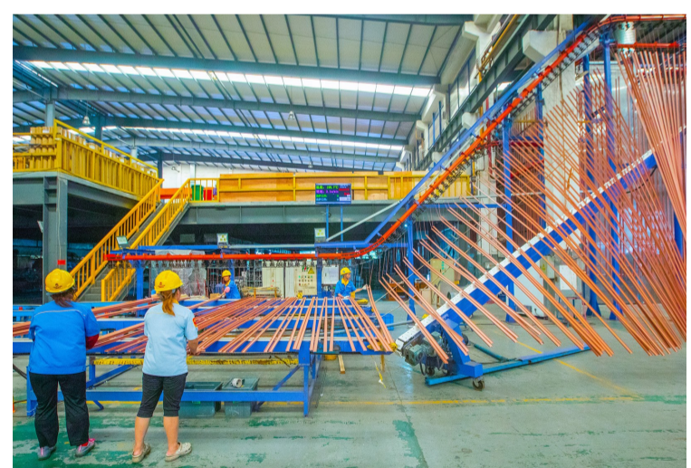
华昌铝材生产车间。
