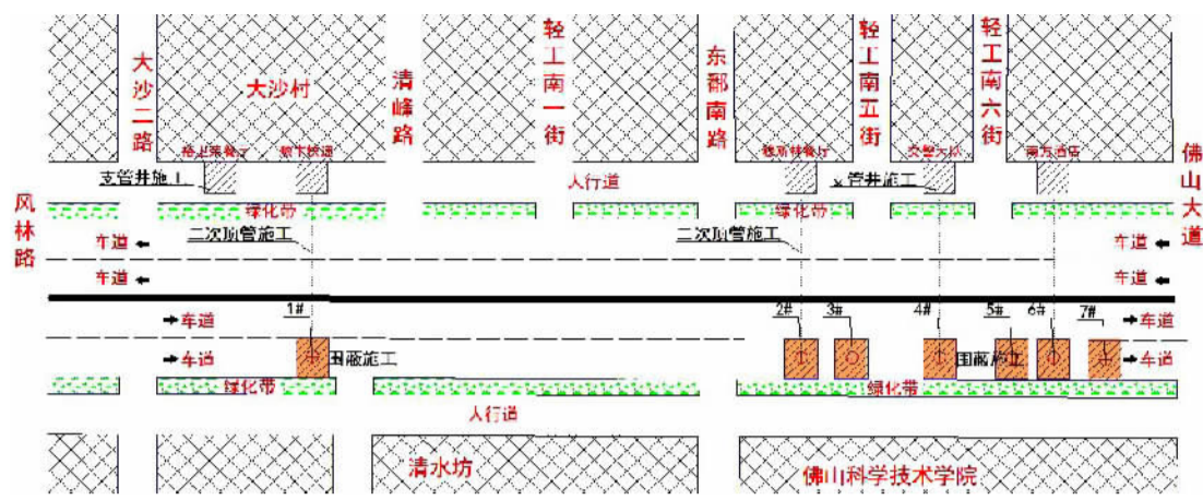
■五峰路围蔽施工示意图。(禅城交警供图)
